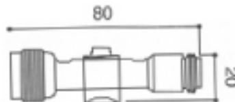
DS-N 尺寸图
