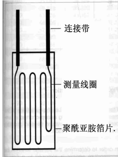
图6. 箔片封装的铂电阻温度传感器 薄膜式铂电阻温度传感器—PCA, 带连接线
