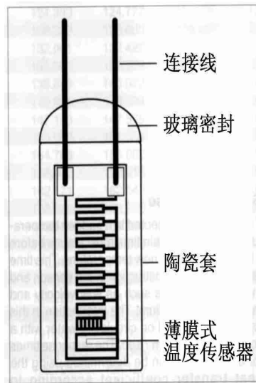
图8. 薄膜式铂电阻温度传感器 带连接线,圆柱形
