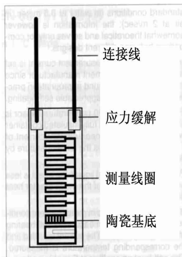
图7. 薄膜式铂电阻温度传感器 带连接线
