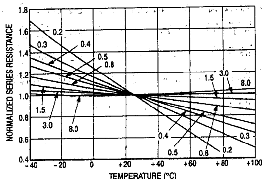
图 2-1 理想温度补偿的归一化串联电阻与温度的关系(不同的 R/R_x 比值)
