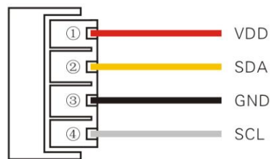
图 1: AM2311 接线图
