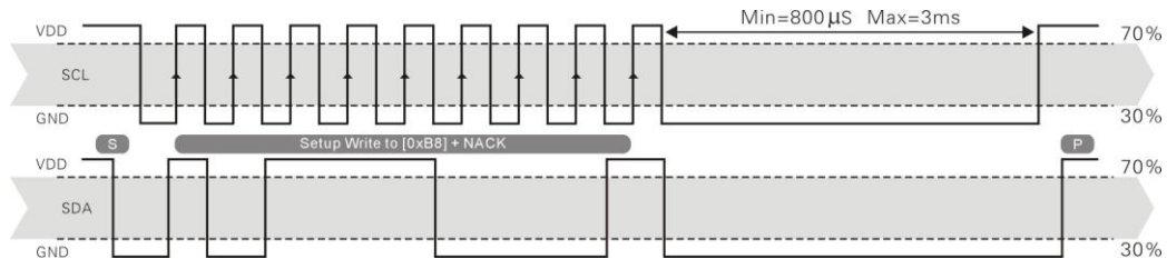
图 14: 唤醒传感器
