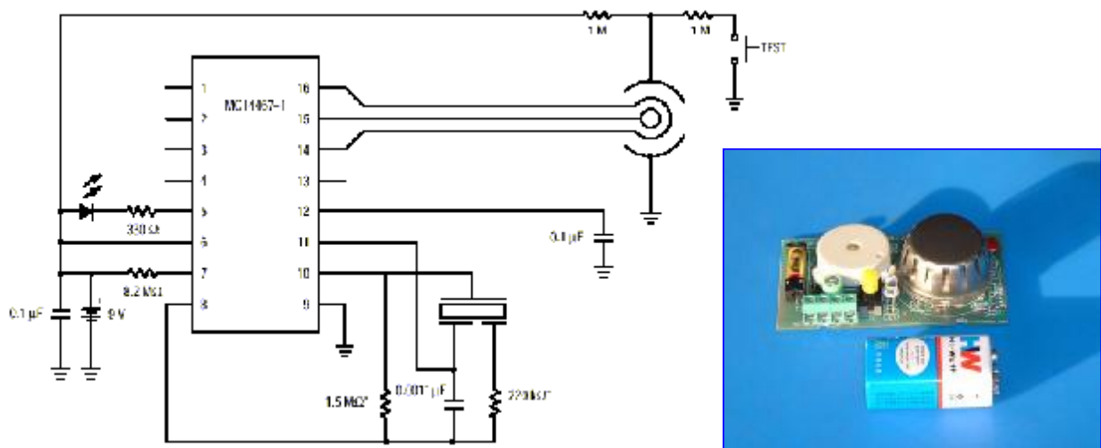
采用 MC14468 的烟雾探测器电原理图
