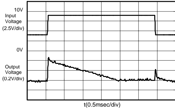
S-8520/1C33MC (Iout:10mA)
