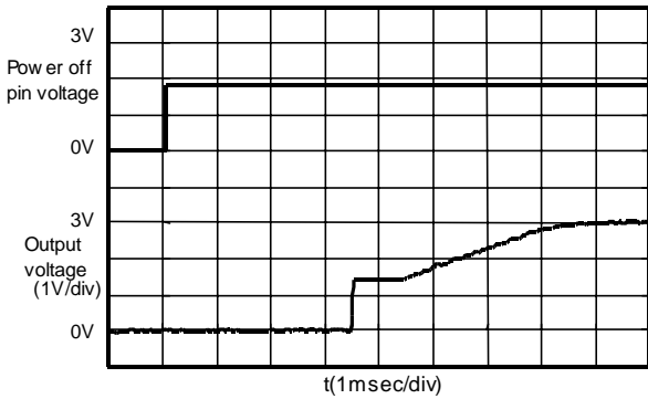
S-8520/1A30MC (Vin:3.6V)
