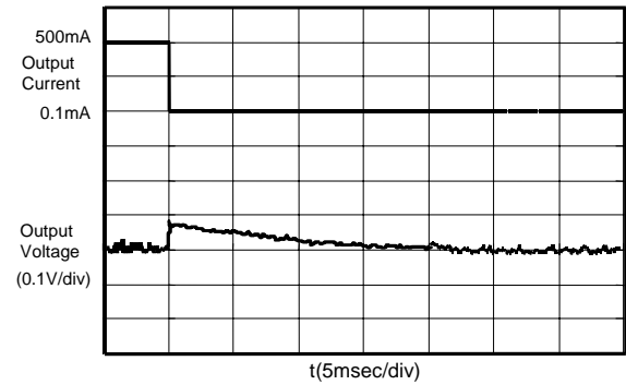
S-8520/1E33MC (Vin:4.0V)
