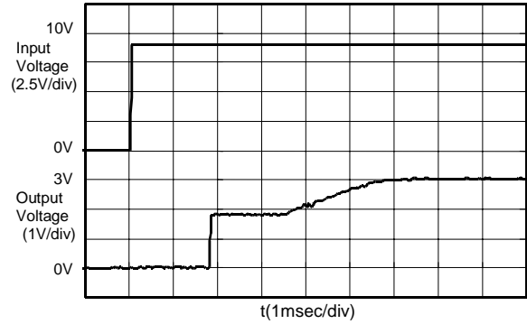
S-8520/1A30MC (Vin:0→9.0V)
