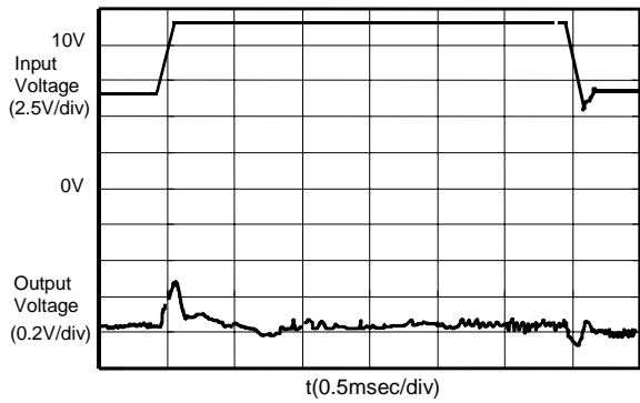
S-8520/1E33MC (Iout:10mA)
