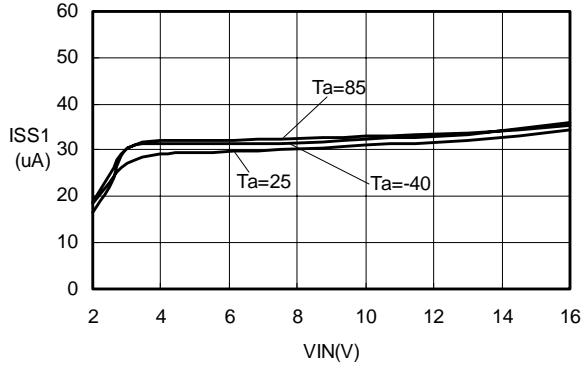
ISS1-VIN S-8520/21(Fosc:300kHz)
