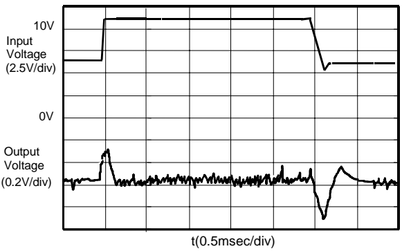
S-8520/1E33MC (Iout:500mA)
