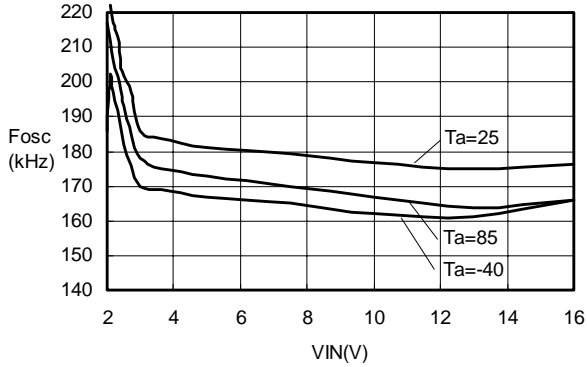
Fosc-VIN S-8520/21(Fosc:180kHz)
