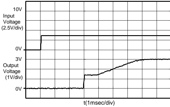
S-8520/1A30MC (Vin:0→3.6V)
