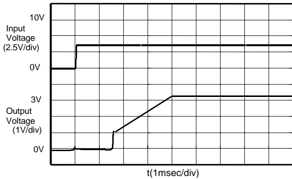
S-8520/1E33MC (Vin:0→4.0V)
