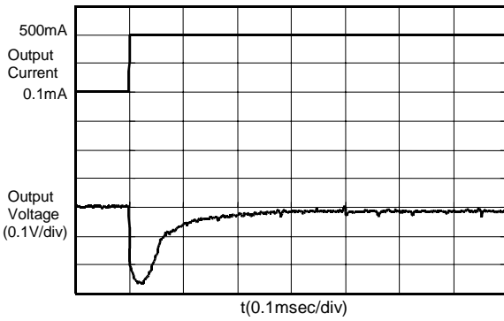
S-8520/1A30MC (Vin:3.6V)
