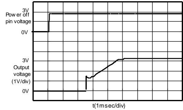
S-8520/1E33MC (Vin:9.0V)
