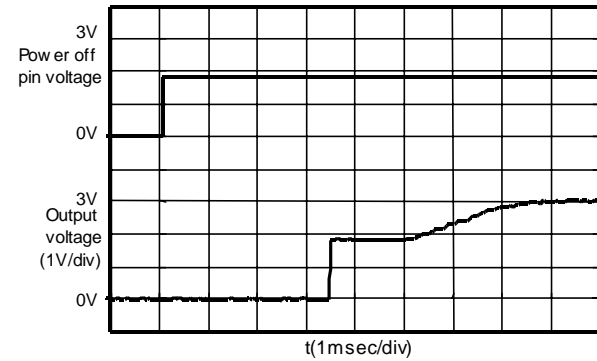
S-8520/1A30MC (Vin:9.0V)
