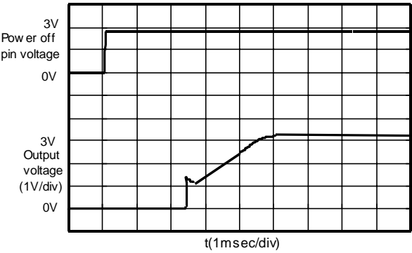
S-8520/1E33MC (Vin:4.0V)
