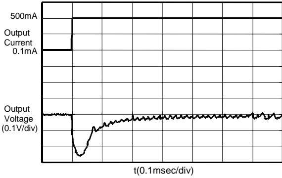
S-8520/1C30MC (Vin:3.6V)
