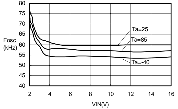
Fosc-VIN S-8520/21(Fosc:60kHz)
