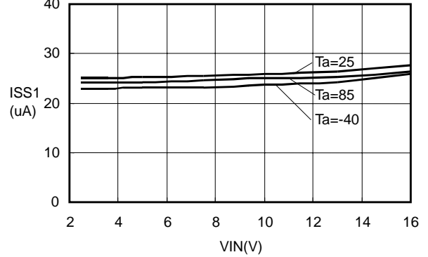
ISS1-VIN S-8520/21(Fosc:180kHz)
