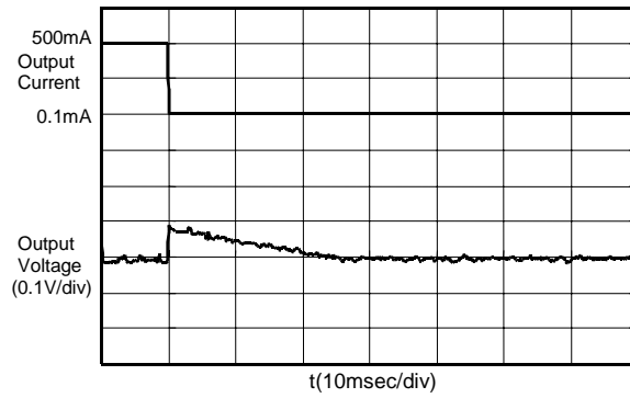
S-8520/1A30MC (Vin:3.6V)
