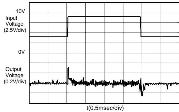
S-8520/1A30MC (Iout:500mA)
