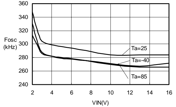
Fosc-VIN S-8520/21(Fosc:300kHz)
