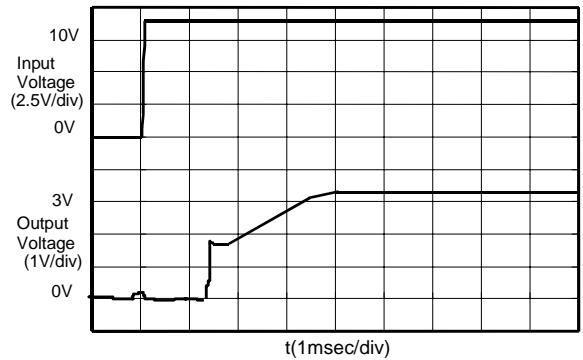
S-8520/1E33MC (Vin:0→9.0V)
