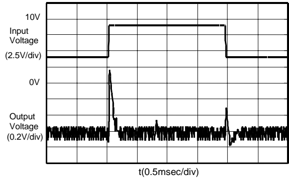
S-8520/1C33MC (Iout:500mA)
