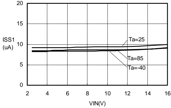
ISS1-VIN S-8520/21(Fosc:60kHz)
