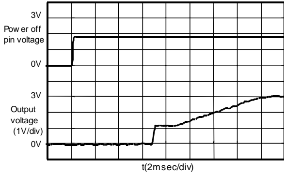
S-8520/1C30MC (Vin:3.6V)
