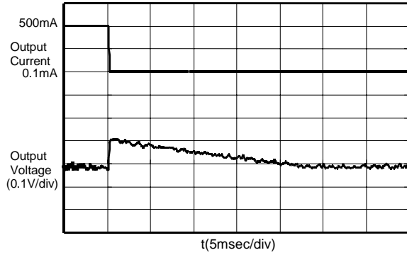
S-8520/1C30MC (Vin:3.6V)
