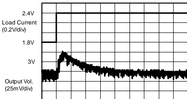
t (100µsec/div)
