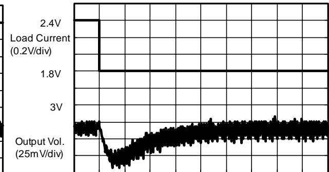
t (100µsec/div)
