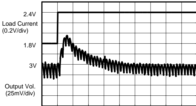
t (100µsec/div)
