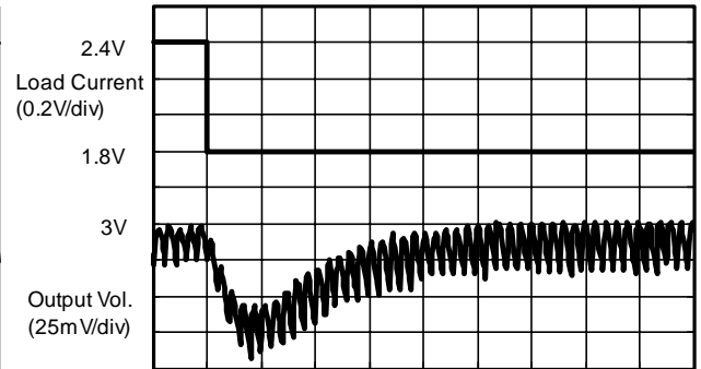
t (100µsec/div)
