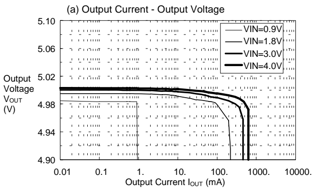
(25)S-8327B50(D75C:47 \mu H,Rb=1k \Omega ,Cb=0.0022 \mu F)
