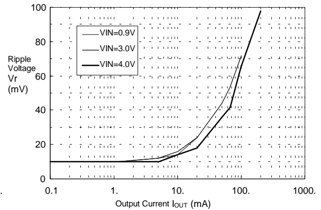
(8)S-8323A50 (CD54:100 \mu H,C OUT :22 \mu F)
