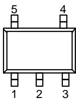
(1) SOT - 23 - 5 Top view
