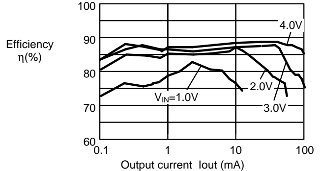
(d) Efficiency - Output current characteristics
