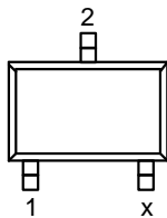
(2) SOT - 23 - 3 Top view
