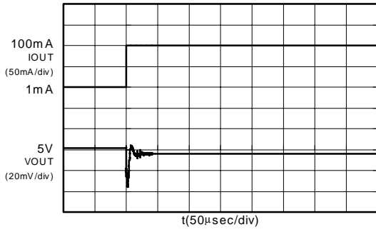
S-816A50AMC (VIN:6V)
