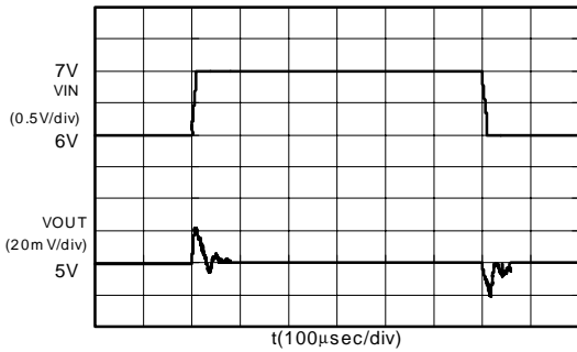
S-816A50AMC (Iout:10mA)
