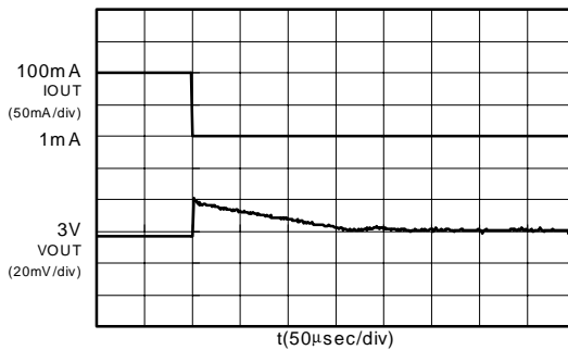
S-816A30AMC (VIN:4V)
