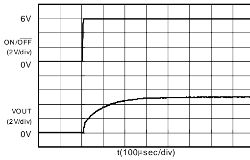
S-816A50AMC (VIN:6V)
