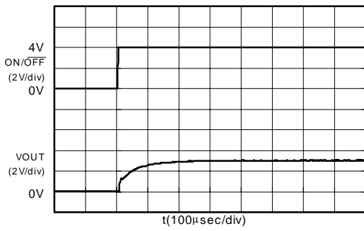
S-816A30AMC (VIN:4V)
