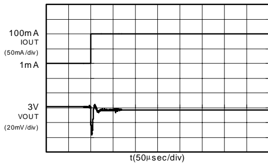
S-816A30AMC (VIN:4V)
