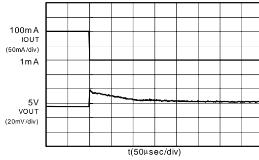
S-816A50AMC (VIN:6V)
