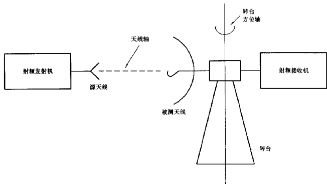
图4 辐射图测量框图的例子
