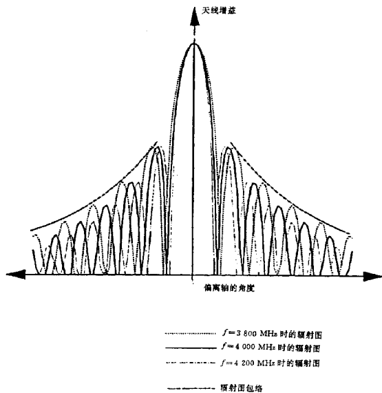
图5 辐射图及其包络的例子
