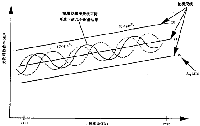
a 用增益基准天线的方法
