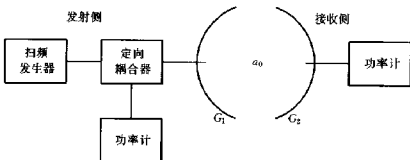
b 增益测量框图
