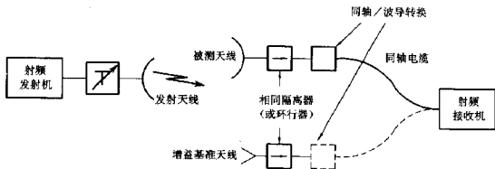
a 用同轴电缆的测量框图
