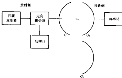
图1 用与增益基准天线比较的方法测量天线增益
