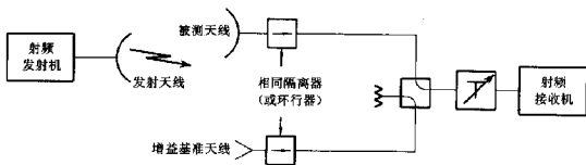
b 用波导的测量框图
