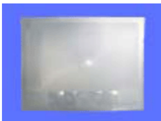
型号: 8204-1(窄角度远距离透镜) 焦距: 25 角度: 10° 距离: 40m 尺寸: 44*56.2
