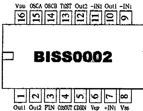
图1 BISS0002外引线连接图
