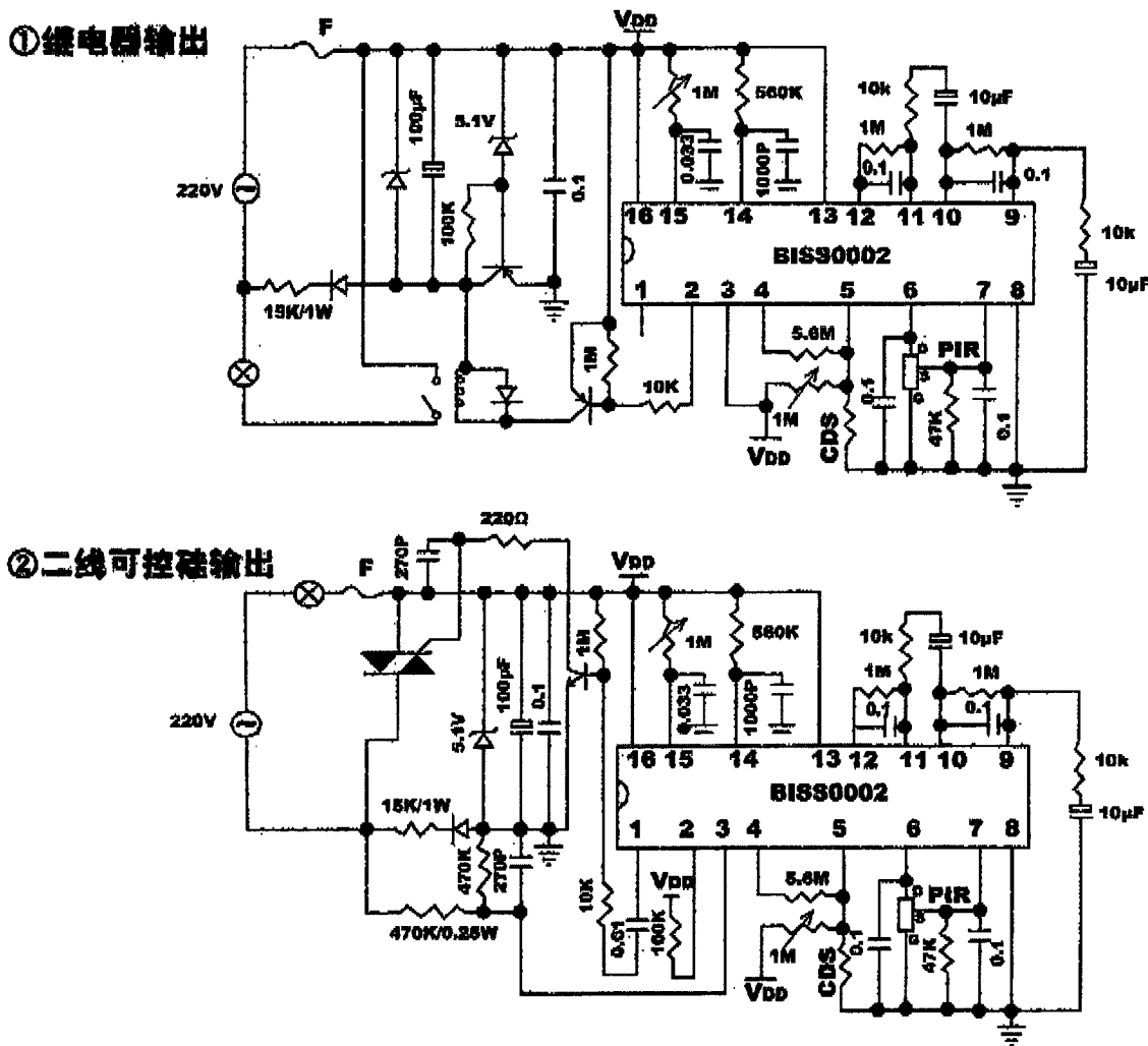
图3 BISS0002应用于热释电红外开关的电路原理图
