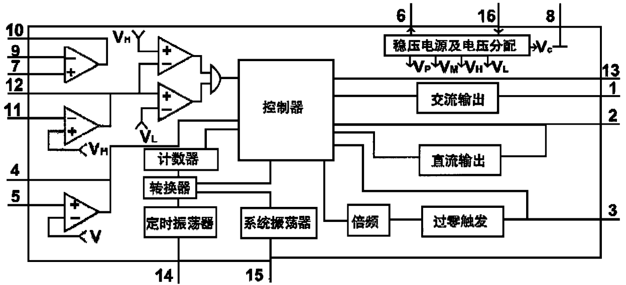
图2 BISS0002原理框图
