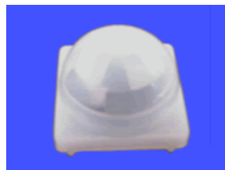
型号: 8002 焦距: 12 角度: 100° 距离: 5m 尺寸: Φ23
