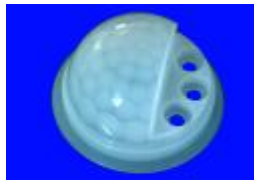
型号: 2091 外径: \Phi 55 内径: \Phi 44 距离: 10m 角度: 120^\circ
