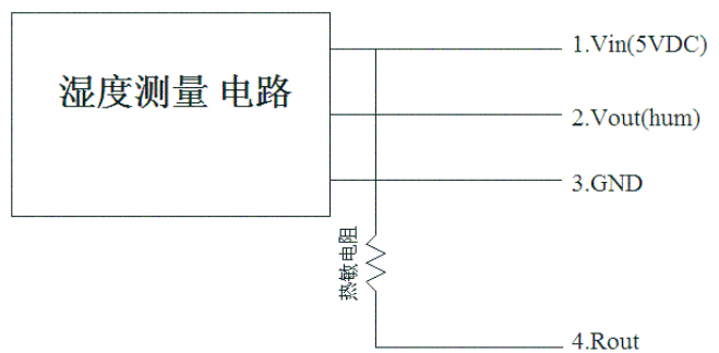
图 2. 接线实例.
