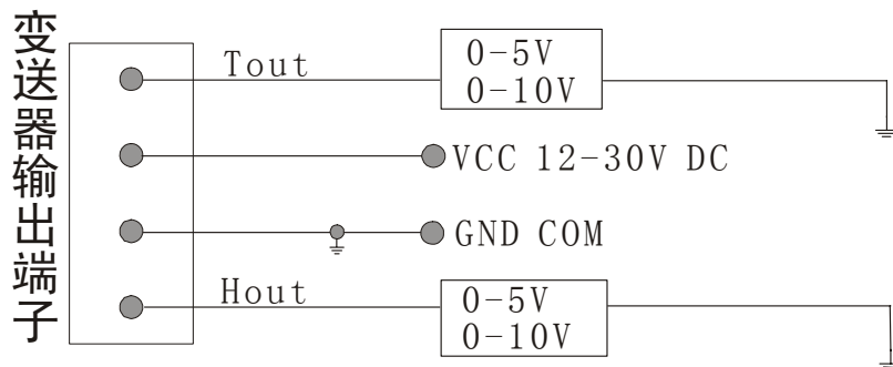
图2:接线图
