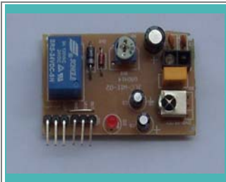
名称：带继电器感应模块 型号：ME001-2
