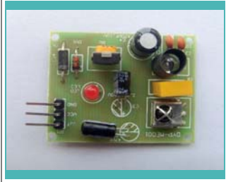
名称：红外感应模块 型号：SSD-ME001-1
