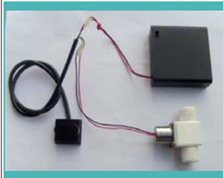
名称： SSD-ME001-1 型号： 水龙头感应模块/洁具感应模块
