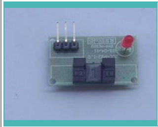
名称：光电开关模块 型号：ME05
