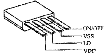
TO92-4L
