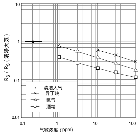
图3 .气敏度特性
