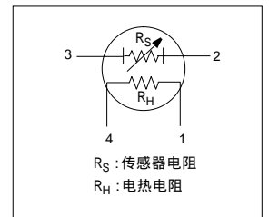
图 1d. 等价回路
