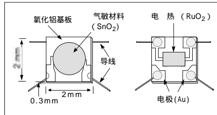
图 1a. 气敏元件
