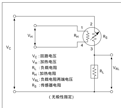
图 2. 标准回路
