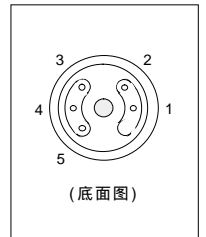
图 1c. 电极端子配置
