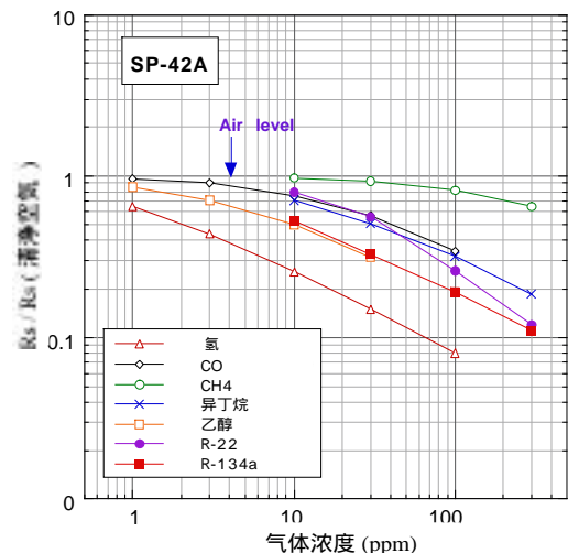
图 3. 气敏特性
