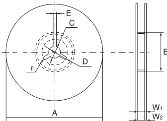
卷盘 Reel
