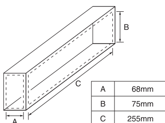
扁平包装 <A21F · A22F> Ammo pack <A21F-A22F>
