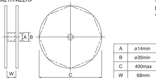
卷盘包装 <A21R · A22R> Reel <A21R-A22R>
