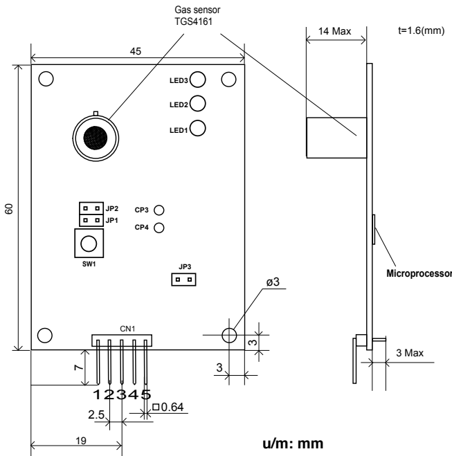
CDM4161 dimensions
