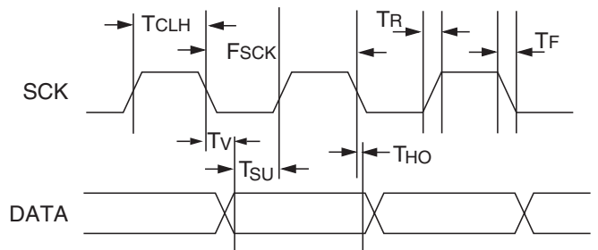
图 9 时序图
