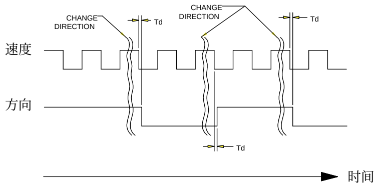
输出定时图
